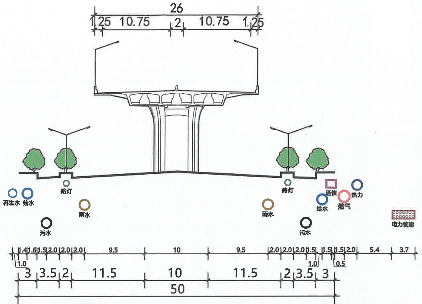
(五三连接线调整前) B2-B2道路横断面 (主干路)
