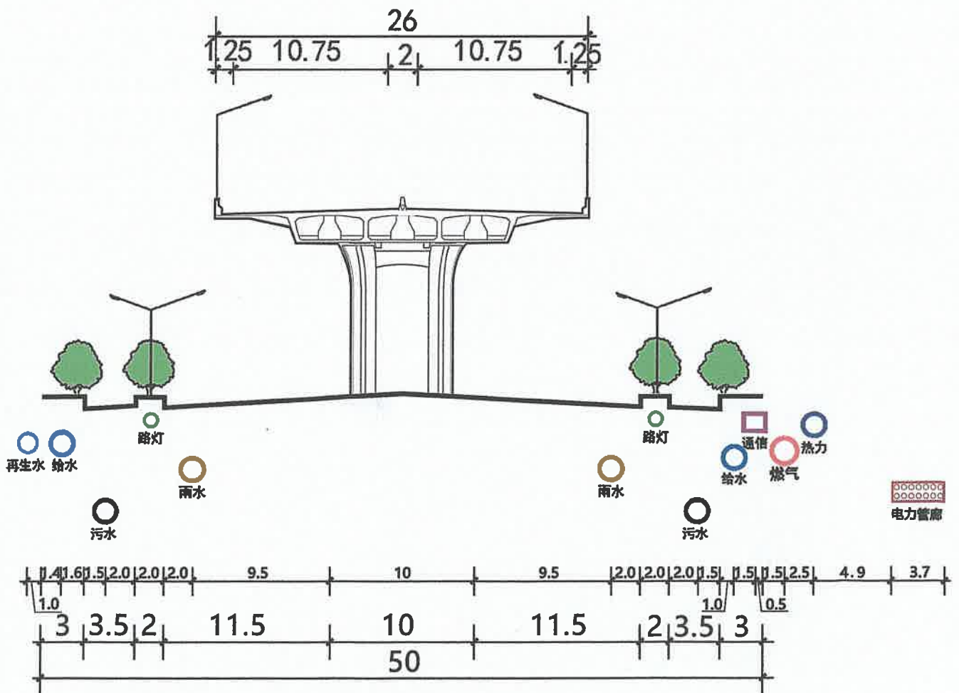
(五三连接线调整后) B2-B2道路横断面 (主干路)
