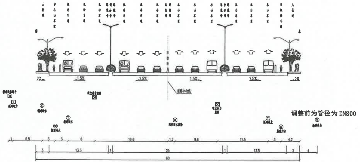
查干沐沁大街管线综合标准横断面图 K4+940.5~K5+320 1:250
