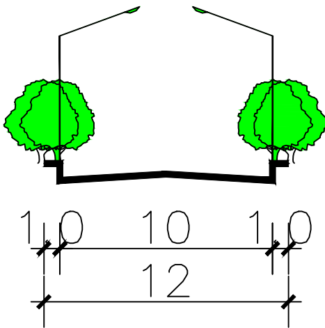
A-A 道路横断面
